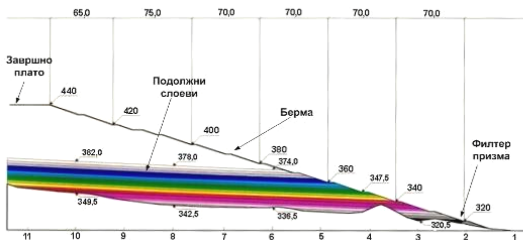
Слика бр.ИИ-11: Пресек на телото на депонијата со завршни косини
