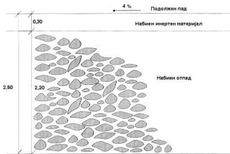
Слика бр.ИИ-10: Пресек на депониски слој
